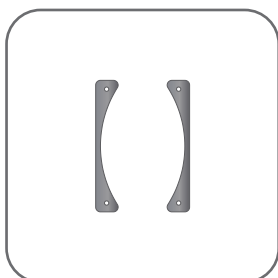
RA730340×2pcs. SPIDER FRAME SPACER FOR 19CM (T=0.5mm) スパイダー枠スペーサー T=0.5mm 19CM用
