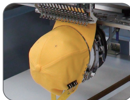
帽子枠
