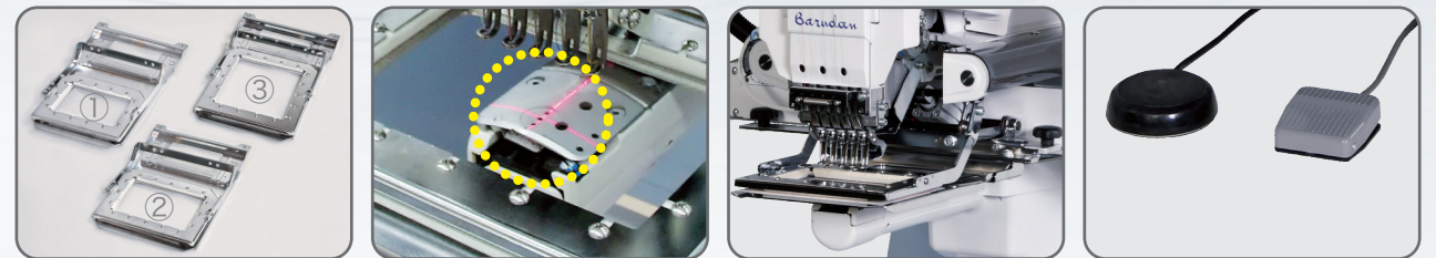
クランプ替枠3種※ レーザーマーカー(クロス) クランプ元枠フレーム フットペダル ※ V250 モデルは ①70 mm × 120 mm ②90 mm × 140 mm ③140 mm × 120 mm のうち 1つ選択
