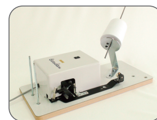
下糸巻き機 (BN-IIIe)
