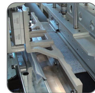
三ッ折部
