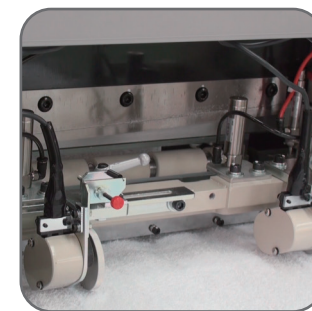
カッター部
